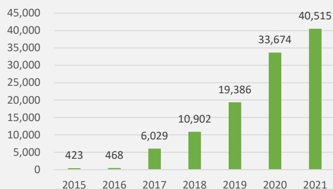
2015年至2021年臺北市太陽光電裝置容量 (單位:瓩)
